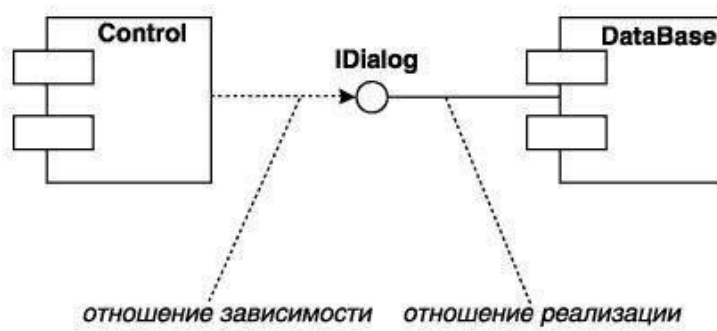
Рисунок 8. Диаграмма компонентов
