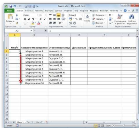
Рисунок 18. Автозаполнение
