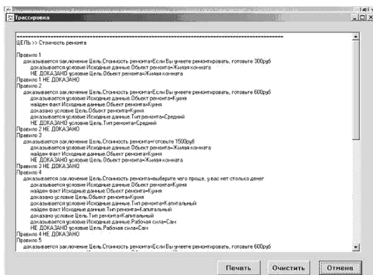
9 Объяснительная компонента экспертной системы (рисунок 5)
