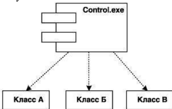
Рисунок 10. Зависимости
