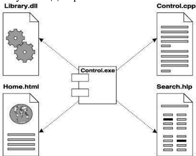
Рисунок 9. Зависимости
